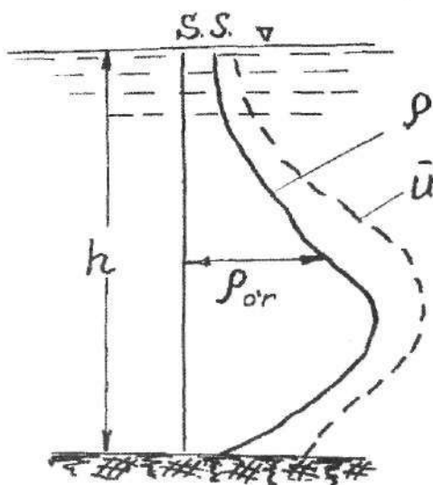
2.27-rasm. Oqiziqalarni chuqurlik bo'yicha taqsimlanishi:
