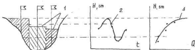
2.23-rasm. Suv sathining oʻrtacha kunlik hisobini aniqlash chizmasi
