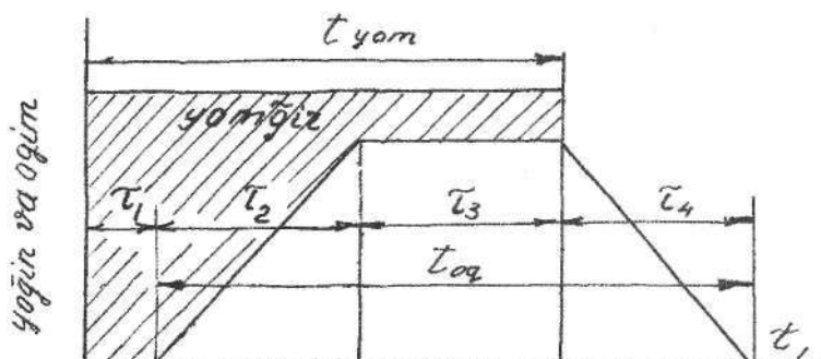
1.9-rasm. N.E.Dolgov tajribasi bo'yicha yomg'ir suvlaridan yer yuzasida oqim hosil bo'lish davrlari
