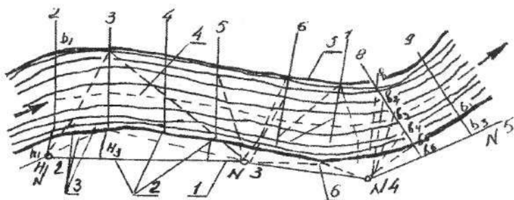
2.8-rasm. Suvning chuqurliklarini ko'ndalang kesimi bo'yicha o'lchash:
