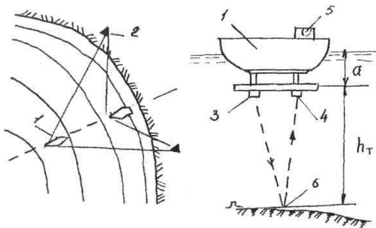
2.7-rasm. Exolot yordamida chuqurliklarni o'lchash:
