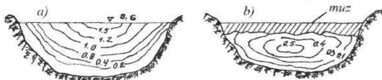
2.13-rasm. Izotaxa chiziqlarining ko'rinishi (a – ochiq havzada; b – muz ostida)
