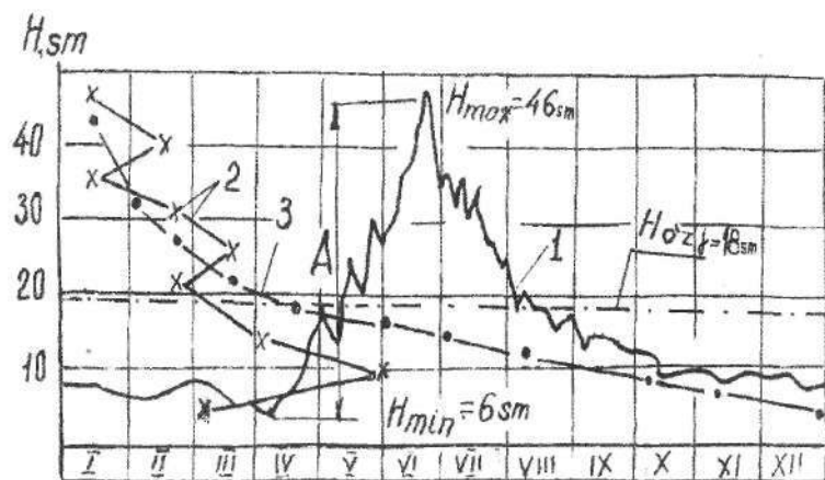
2.4-rasm. Suv sathining yillik grafigi:
